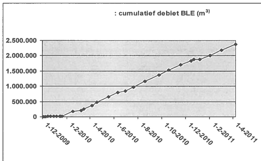
Grafiek 1: Ontrokken volume (m 3 ) bodemlucht (cumulatief)
