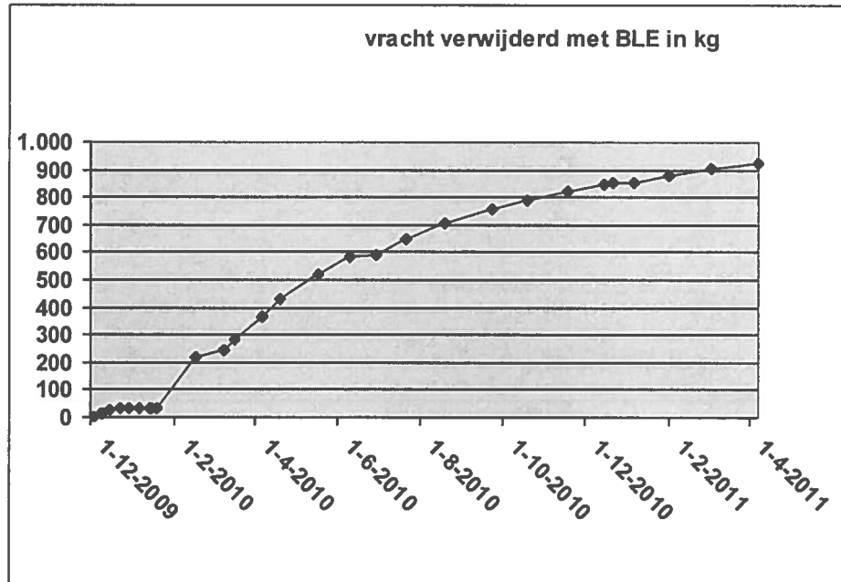
Grafiek 3: Berekende verwijderde vracht aan PER via de onttrokken bodemlucht (cumulatief)
