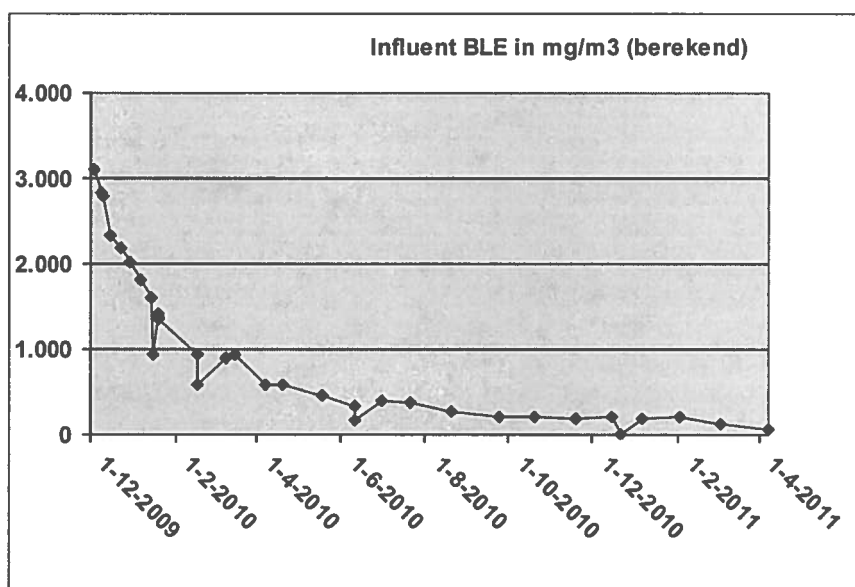
Grafiek 2: Verloop influent concentratie PER in onttrokken bodemlucht
