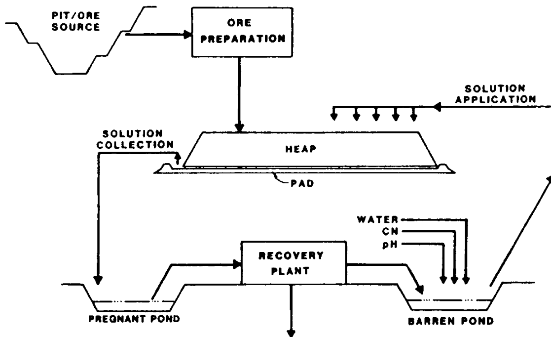
Fig. 2. Schematische weergave van heap leaching.
