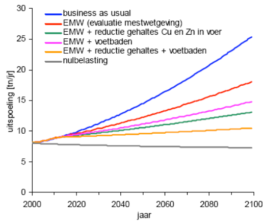
Figuur 3.2 Scenarios voor de ontwikkeling van koperuitspoeling in Nederland in ton/ha (Bron: Bonten et al. 2009, Alterra rapport 1818)
