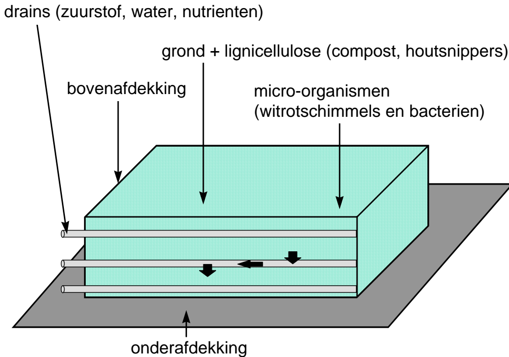
Figuur 1 Voorbeeld van de technische voorzieningen bij een civieltechnisch werk
