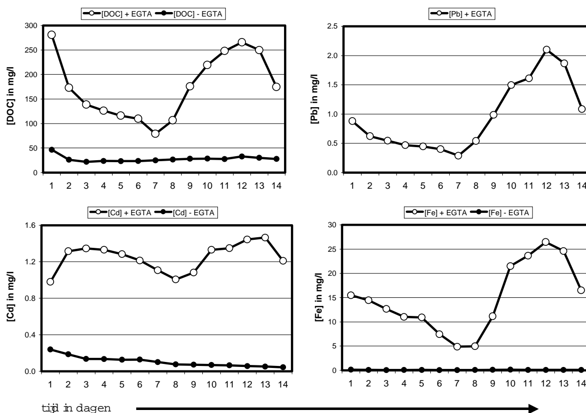
Figuur 8: De invloed van toevoeging van EDGA (=EGTA) op de uitspoeling van DOC, Pb, Cd en Fe, gemeten als concentratie in het drainwater tegen de tijd in lysimeters op de Sinderhoeve.
