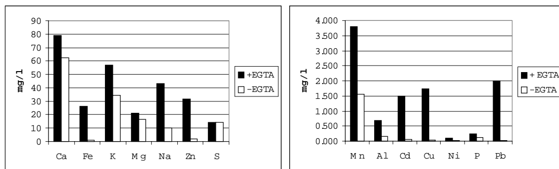
Figuur 7: De invloed van toevoeging van EDGA (=EGTA) op de aanwezigheid van macro-elementen en zware metalen in het drainwater van Budel-grond in lysimeters op de Sinderhoeve; maximale waarden.
